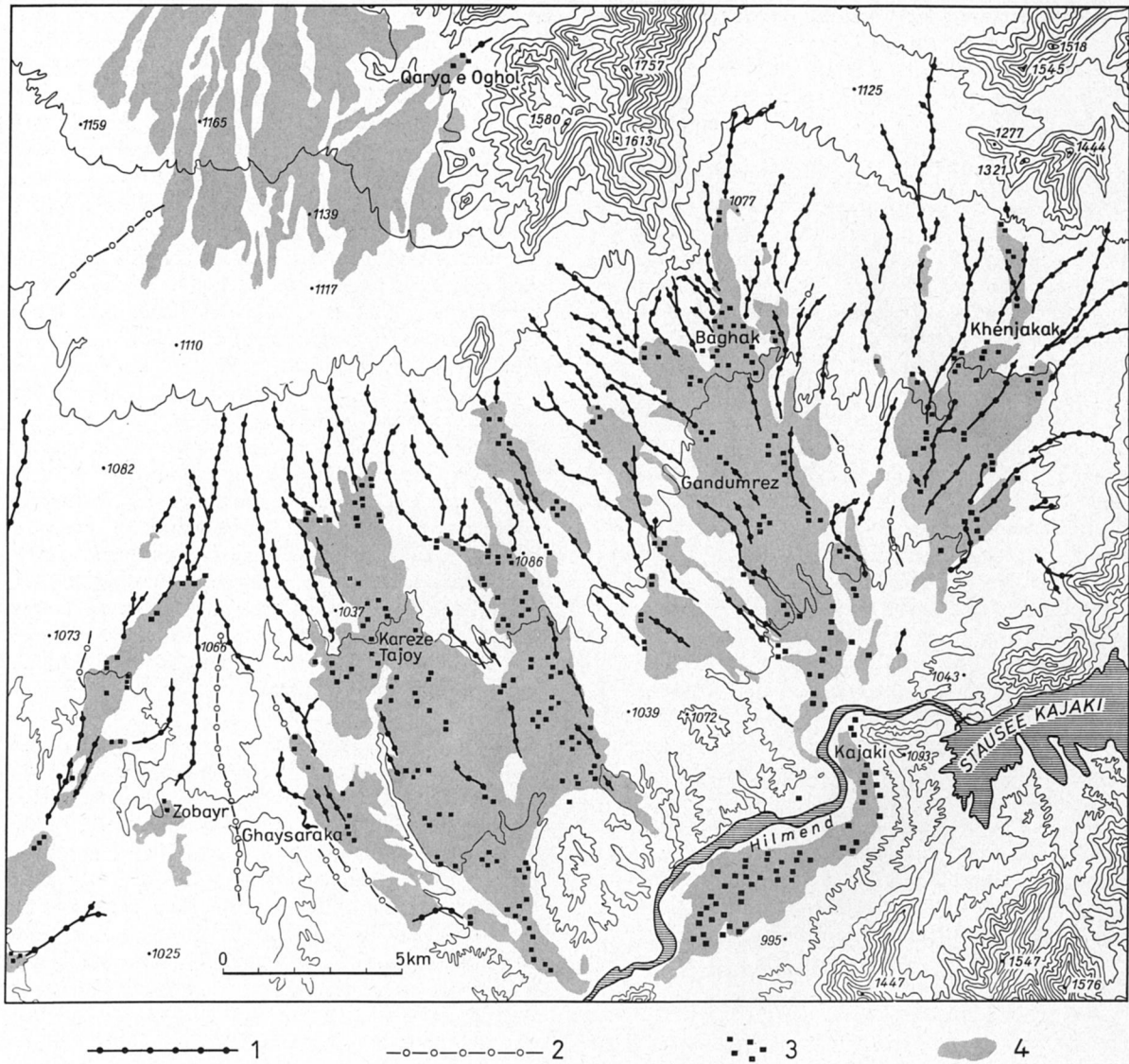
Abb. 1: Kareze-Abfolgen am mittleren Hilمند bei Kajaki/Afghanistan
