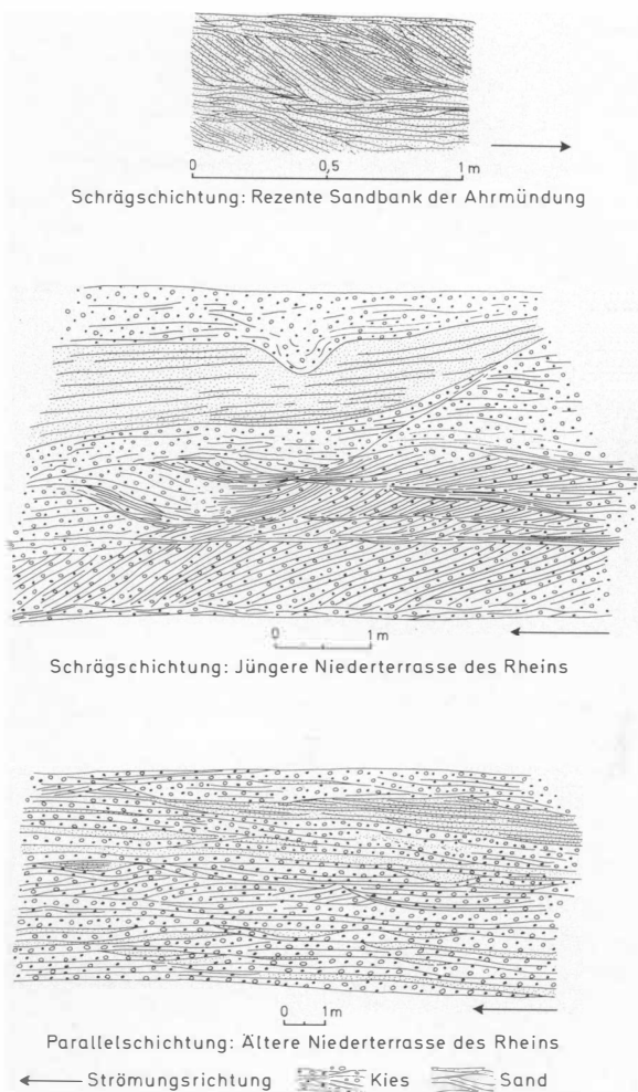
Abb. 4: Schichtungsmerkmale verschiedener Flußsedimente im Ahrmündungsgebiet. Oben : Schrägschichtung von Sanden, Ahrmündung am 5. 10. 1977. Mitte : Schrägschichtung der jNT-Sedimente des Rheins südlich von Remagen; die Sande und Fein- bis Mittelkiese wurden von einem verzweigten Rheinlauf transportiert und sedimentiert. Unten : Parallelschichtung der äNT-Sedimente des Rheins südlich von Sinzig; die Grobkiese und Sande wurden von einem schießend abkommenden Rhein transportiert und sedimentiert
